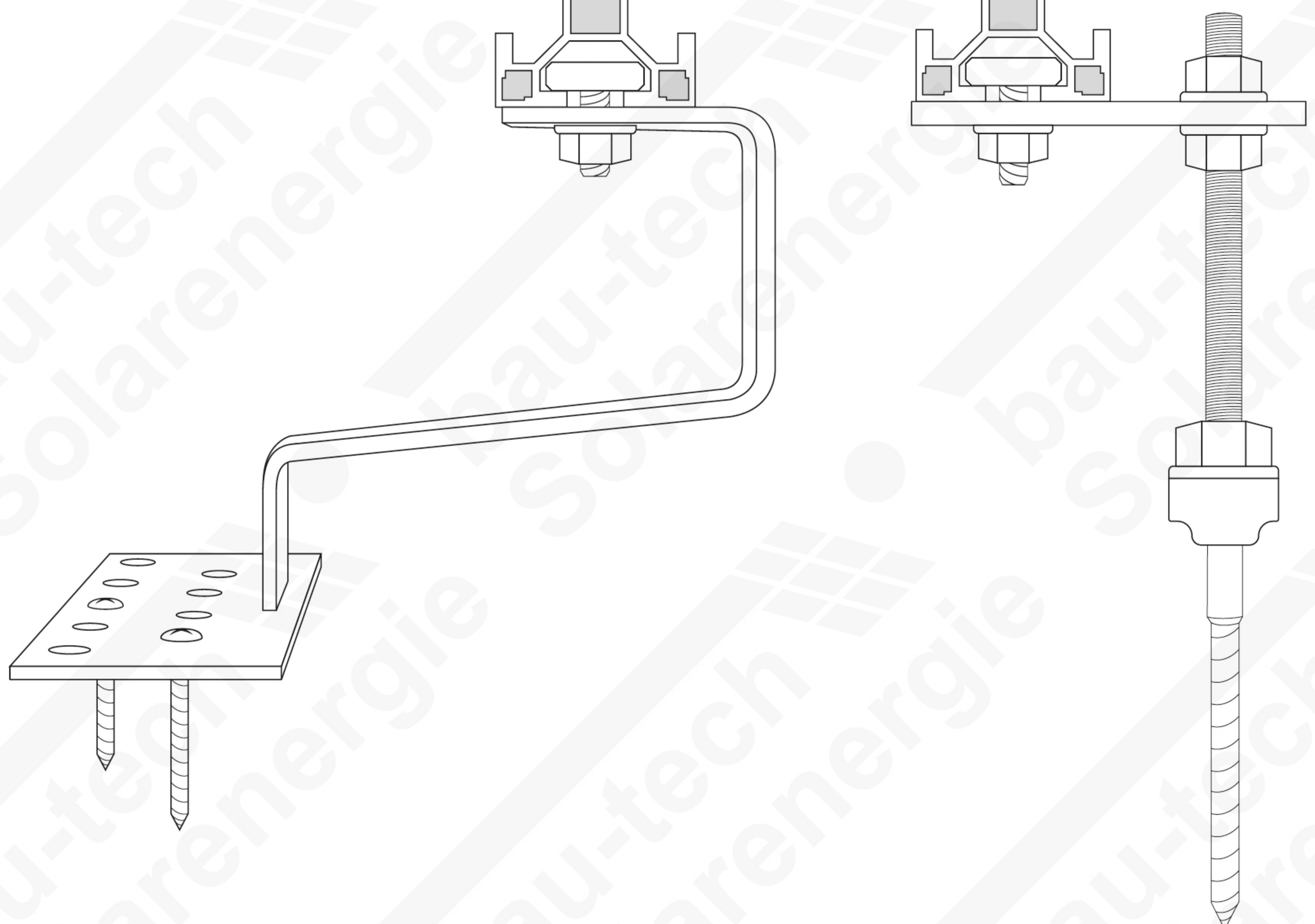
Stockschraube
