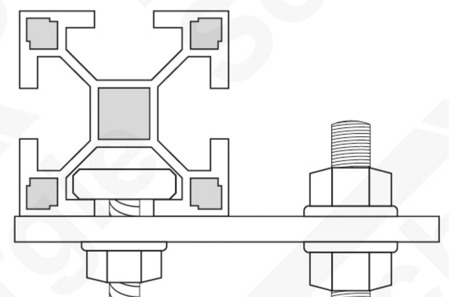
Stockschrauben
