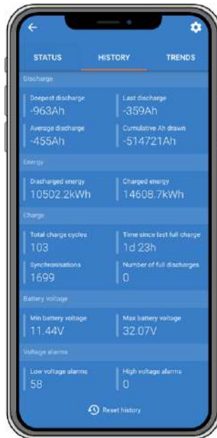
Verlaufsanzeige des Batteriemonitors in der VictronConnect App.
