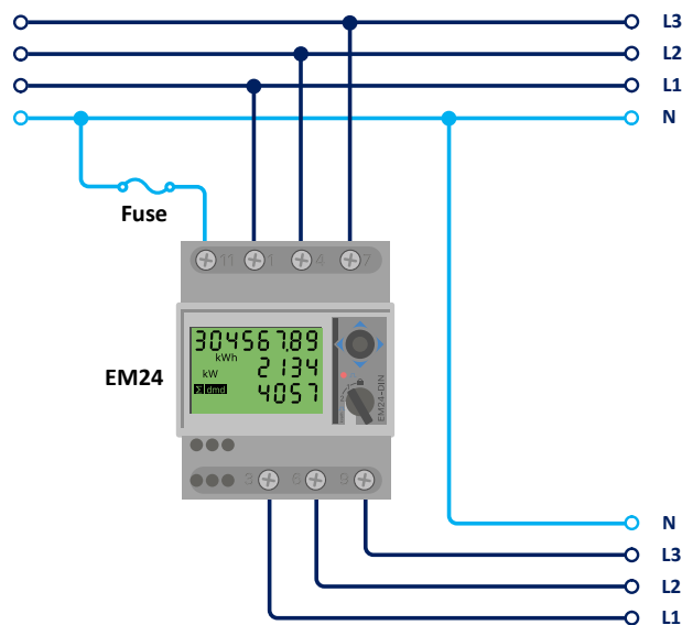
EM24 3-Phasen-Verkabelung
