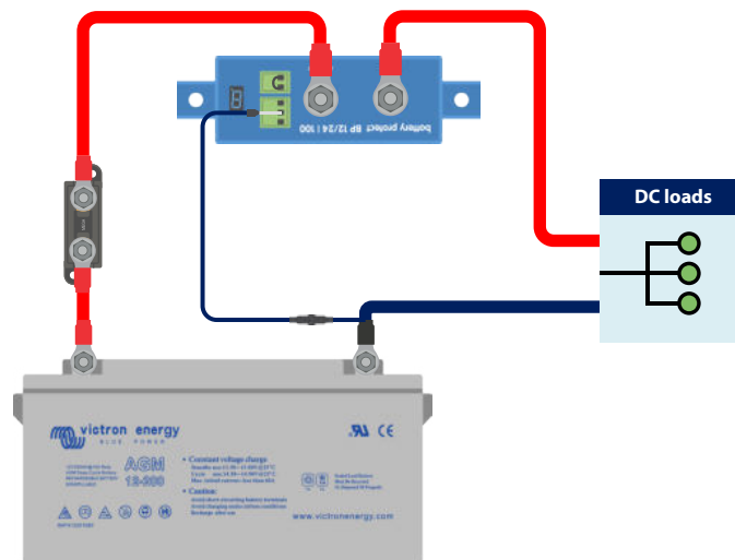
BatteryProtect in einem einfachen System mit einer Drahtschleife zwischen den beiden Pins der Klemme zum ferngesteuerten Ein-/Ausschalten (Werkseinstellung)
